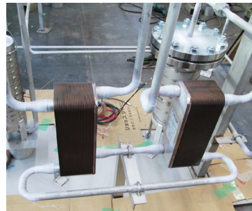
ヘリウムガス冷却装置
