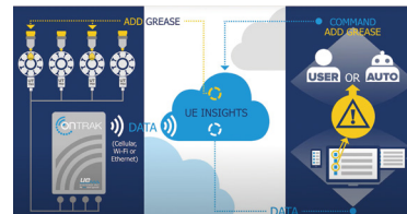
ONTRAK SmartLubeシステム構成図
